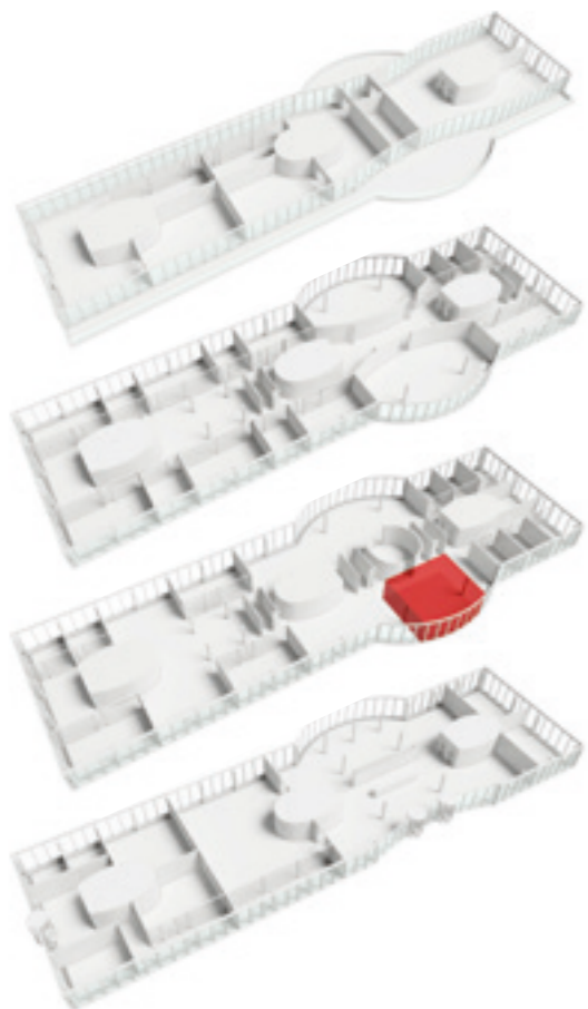
ABSTIMMUNG / COORDINATE
